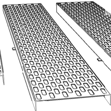
Hullrist til sau, 330 x 2400 mm Byggehøyde 50 mm Varenummer 1050002
