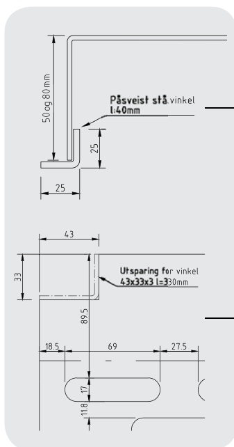
Hullrist til sau, 330 x 2000 mm Byggehøyde 50 mm Varenummer 1050001
